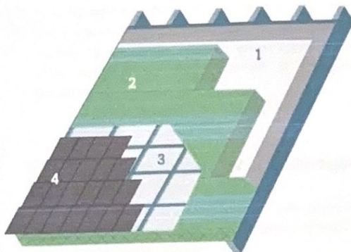
1. Damperscreen | 2. Isolatie | 3. Onderdak | 4. Dakbedekking
