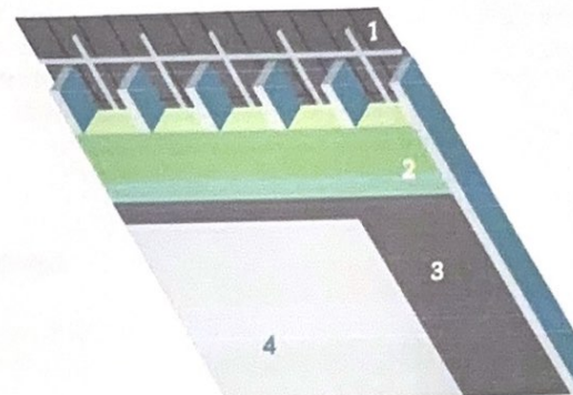
1. Onderdak | 2. Isolatie | 3. Damperscreen | 4. binnenafwerking
